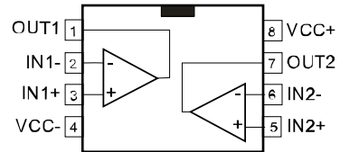
SO8 (TSZ182H1)
