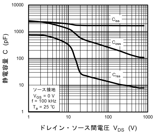
図 8.11 C - V_{DS}
