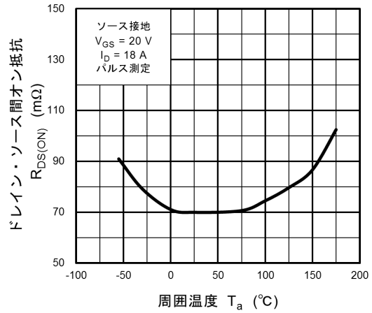
図 8.8 R_{DS(ON)} - T_a
