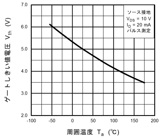
図 8.4 V_{th} - T_a
