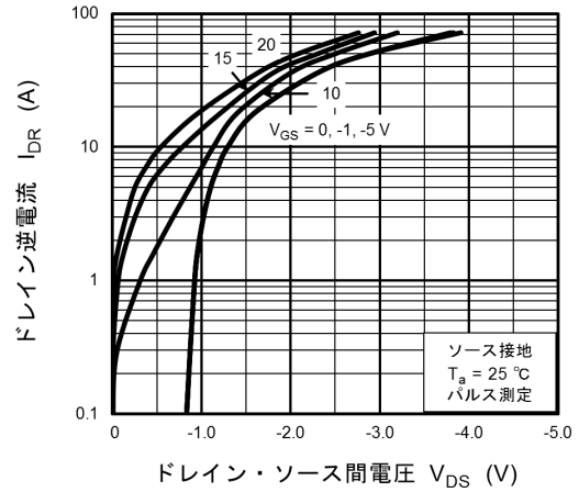
図 8.14 I_{DR} - V_{DS}
