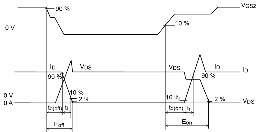
図 6.5.2 タイミングチャート
