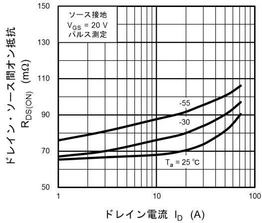
図 8.7 R_{DS(ON)} - I_D
