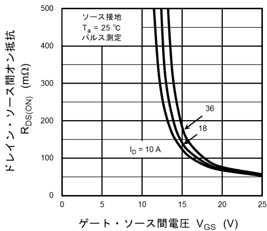
図 8.5 R_{DS(ON)} - V_{GS}
