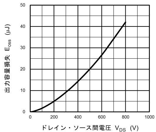
図 8.12 E_{oss} - V_{DS}
