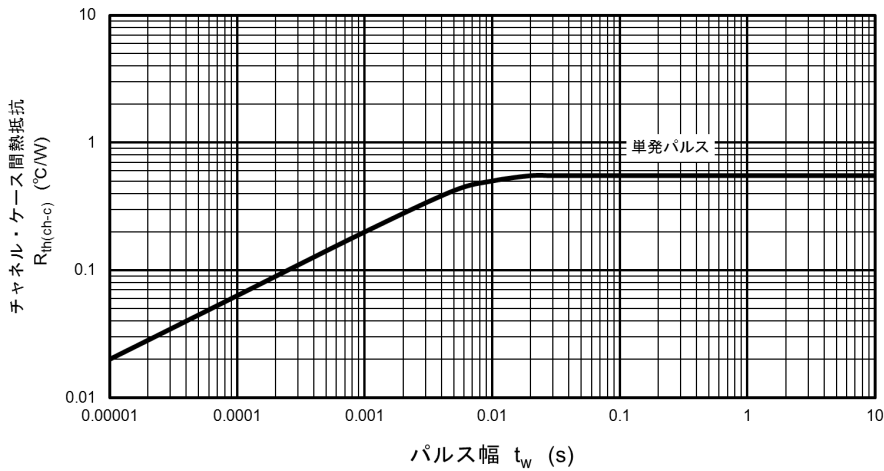
図 8.15 R_{th(ch-c)} - t_w (最大値 (保証値))
