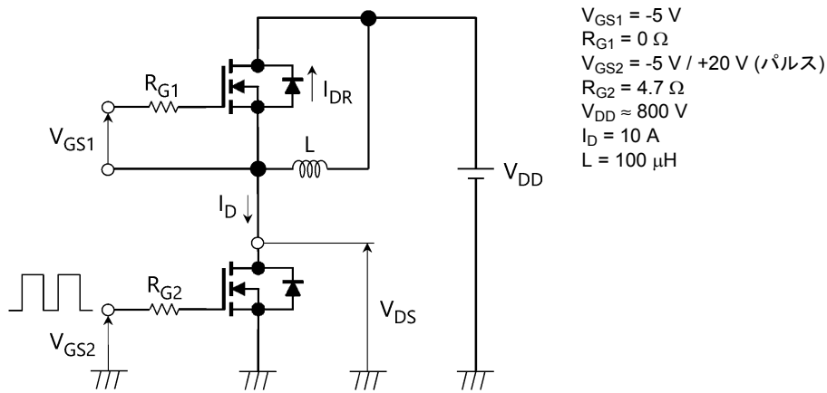
図 6.5.1 スイッチング時間の測定回路
