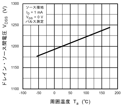
図 8.9 V_{DS} - T_a
